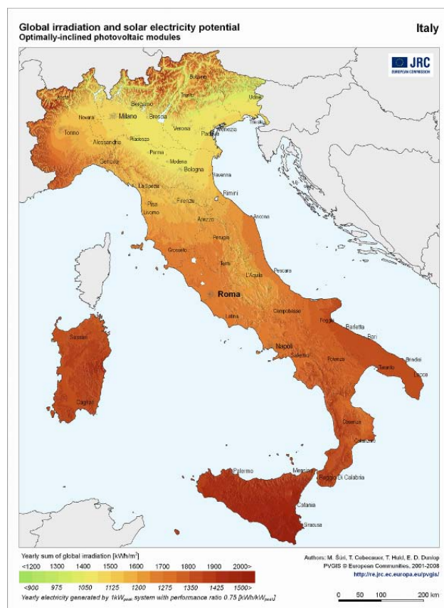
Figura C.1 – Producibilità elettrica annua di un impianto fotovoltaico da 1 kW in Italia
